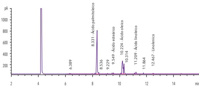
Gráfica. Perfil cromatográfico mediante HPLC del contenido en omegas 3,6,7 y 9 de las bayas del espinillo amarillo.
